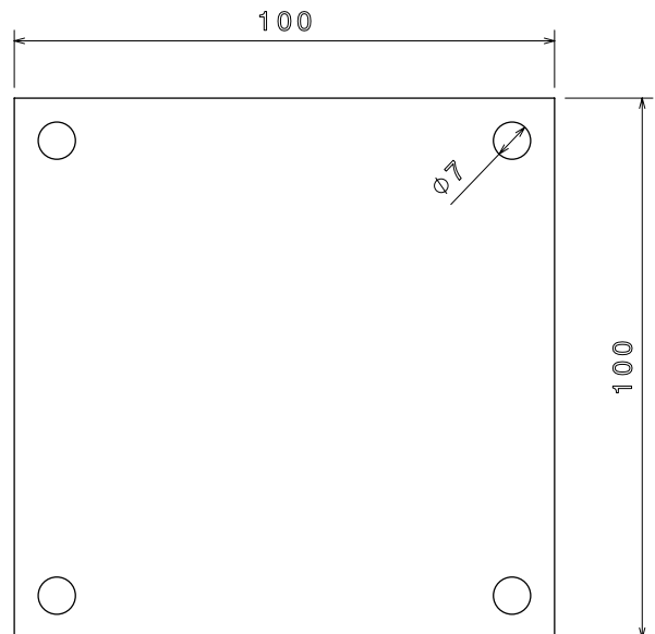
Top view Scale: 1:1
